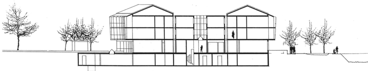
SCHNITT / FASSADE
