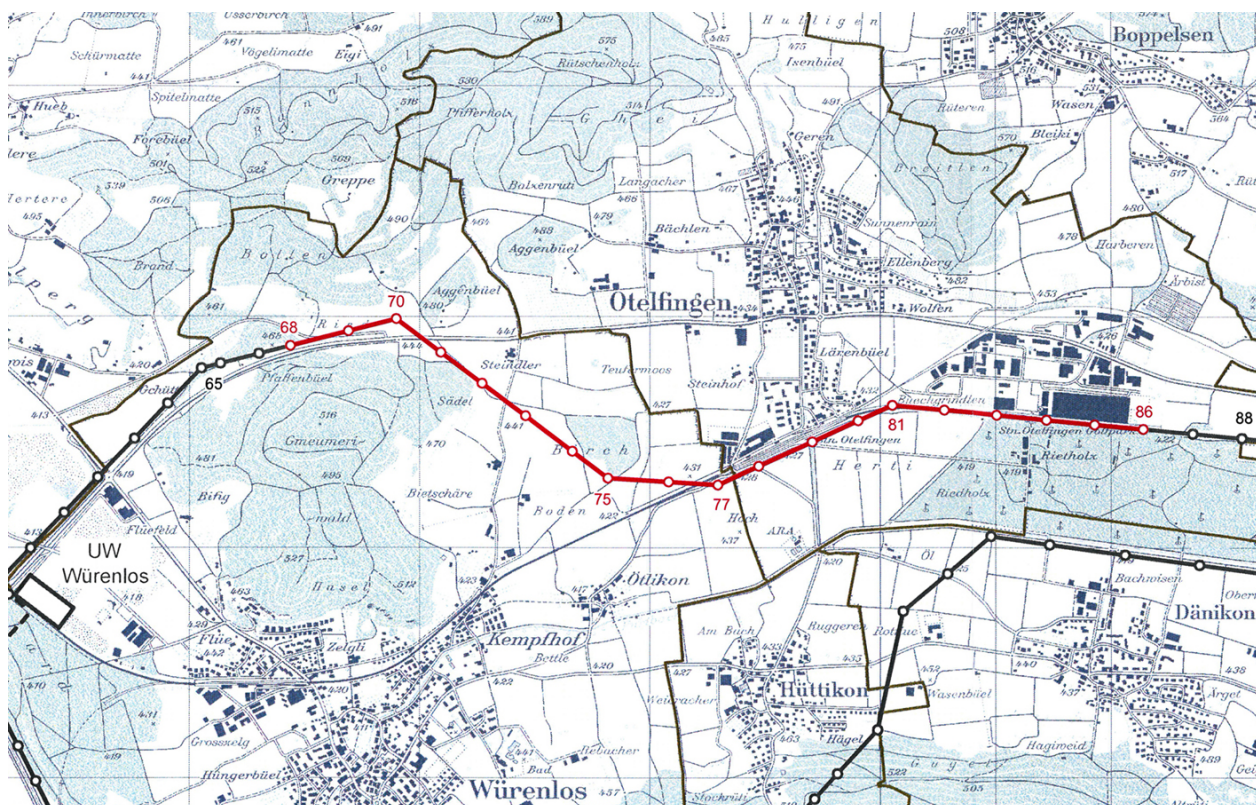
50-kV-Leitung Würenlos-Regensdorf, Abschnitt Mast Nr. 68 bis 86
