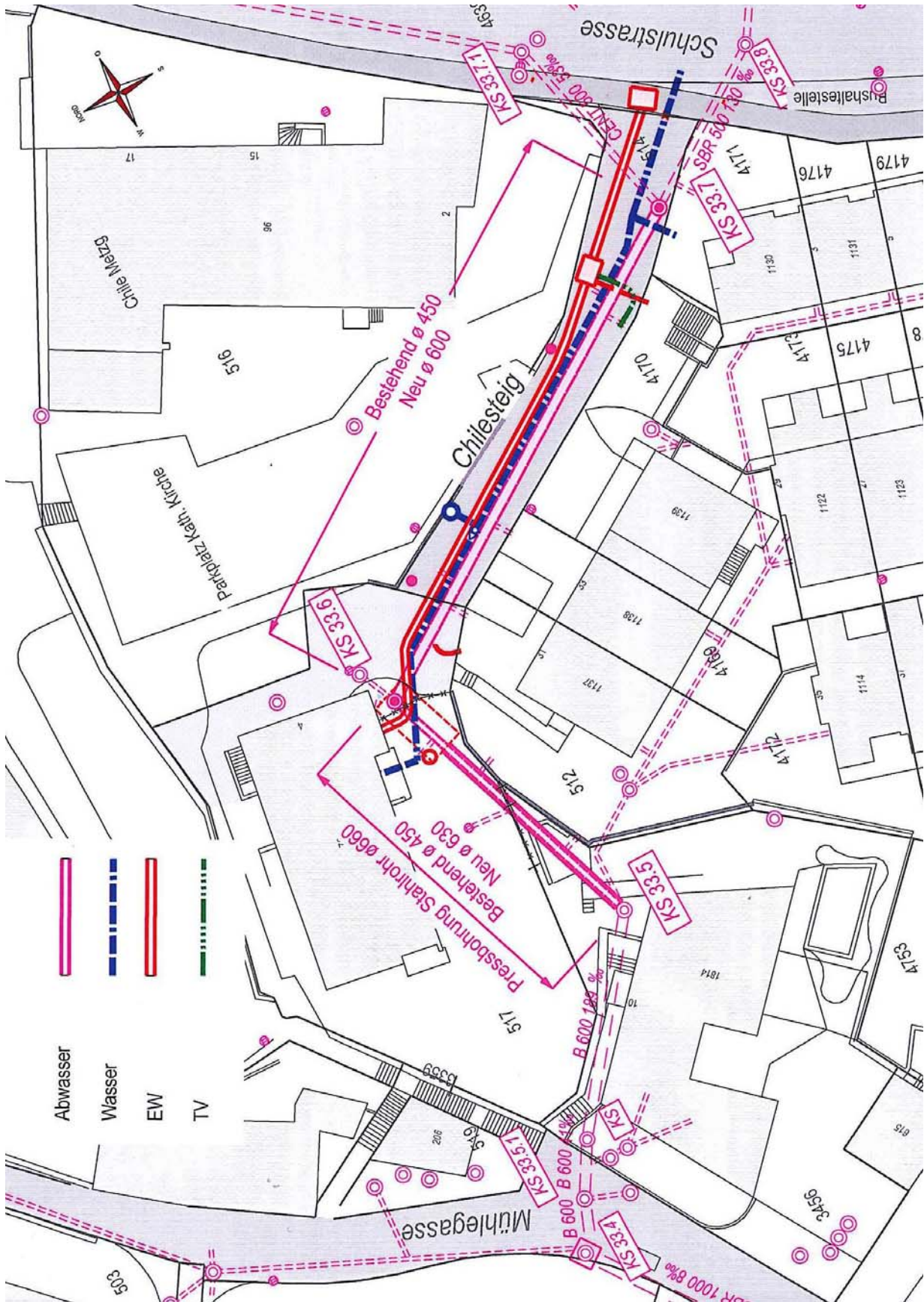
Übersichtsplan über die projizierten Arbeiten
