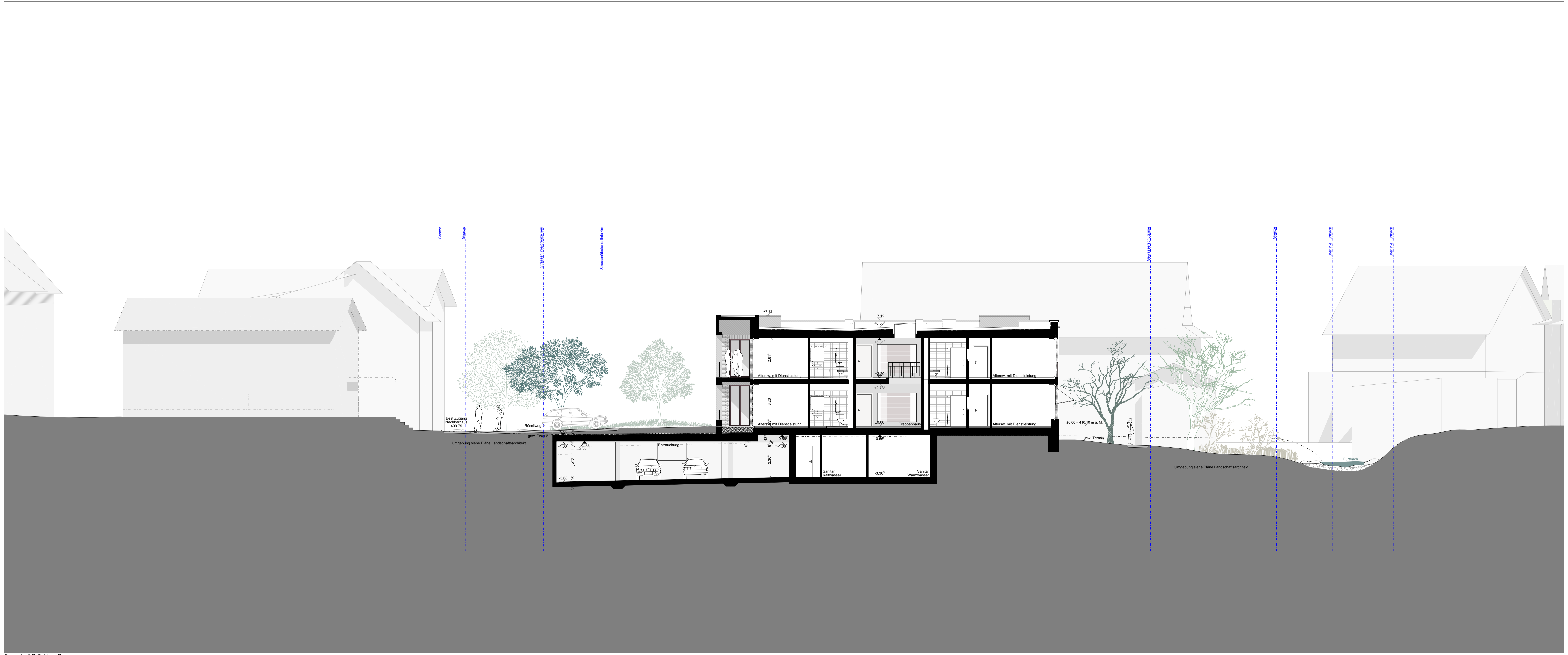
Querschnitt D-D, Haus D
