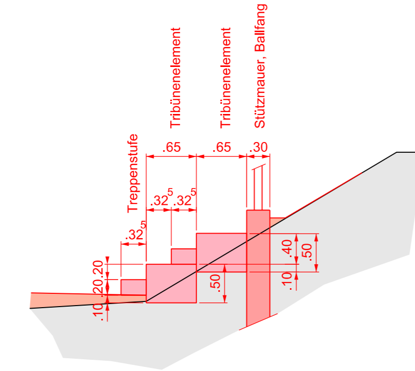
Tribüne in Erdwall integriert, 1:50
